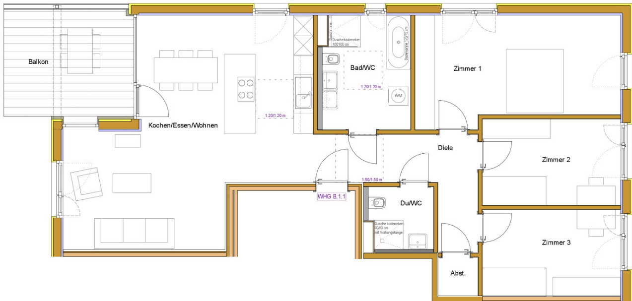
B.1.1_Grundriss
