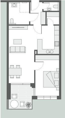
Grundriss
