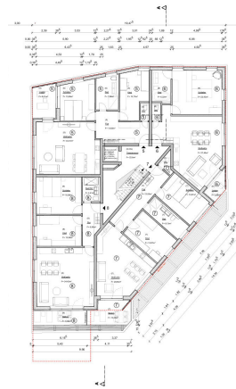
Grundriss OG Whg 5-8
