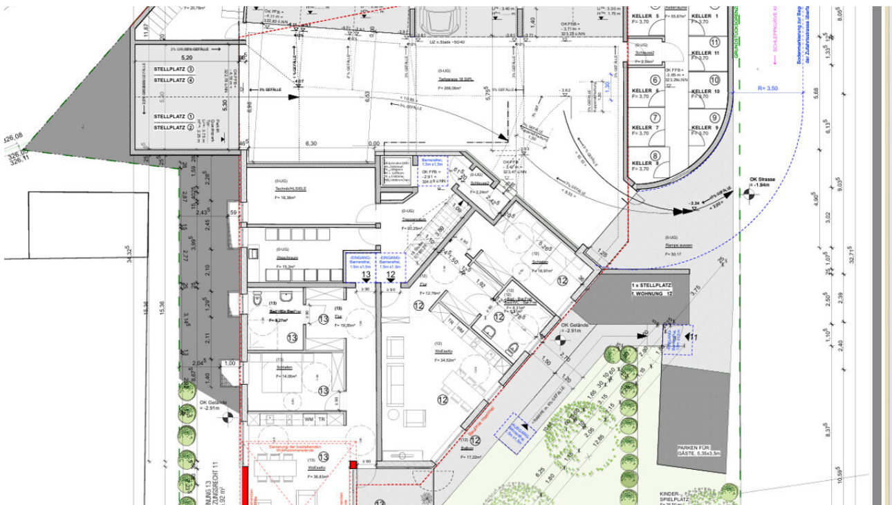
Grundriss UG Whg 12-13 Stellplätze
